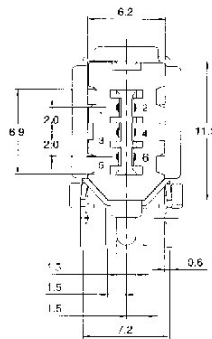
AJ-USB-1394V
