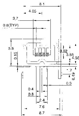
AJ-USB-1394S-4H
