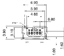
AJ-USB-BS-5B
