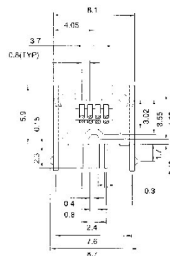
AJ-USB-1394S-4S
